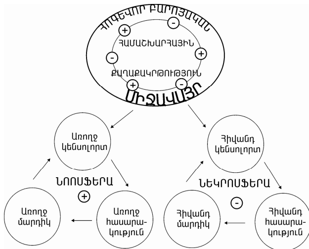
Նոստիքեր և նեկրոսֆերա (ըստ Ն.Ա. Աղաջանյանի, 2001)
